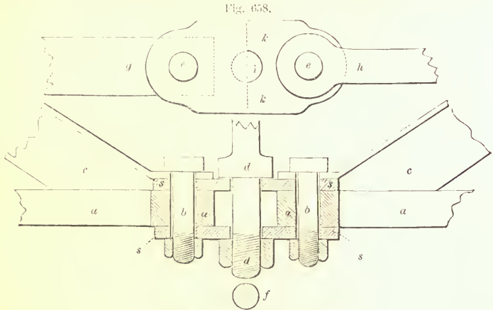
FIG. 658. SECTION AND KING-BOLT.
