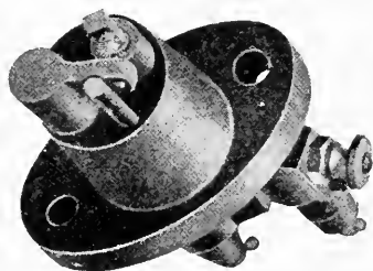
FIG. 306—CONTACT-SPARK IGNITOR
