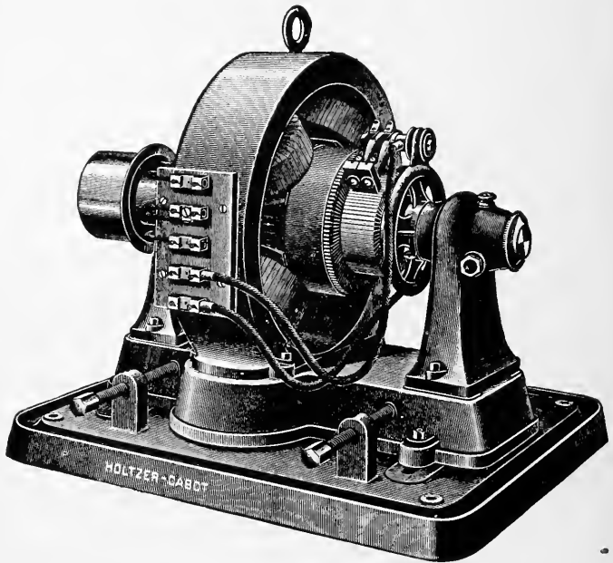
FIG. 367—MULTIPOLAR MOTOR
