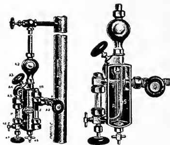
FIG. 279—CYLINDER LUBRICATOR
