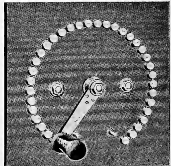
FIG. 349—COMMERCIAL RHEOSTAT
