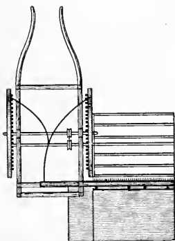
FIG. 105—OGLE'S REAPING MACHINE (ENGLAND, 1822)
