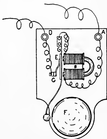
FIG. 354—ELECTRIC BELL
