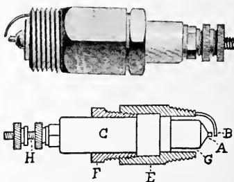
FIG. 307—JUMP-SPARK IGNITOR
