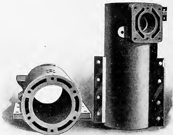
FIG. 290—CYLINDER
