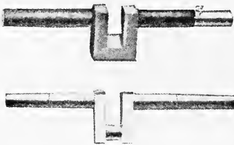
FIG. 294—CRANK SHAFT
