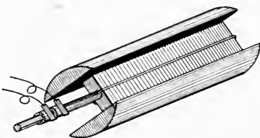
FIG. 358—MAGNETO ARMATURE
