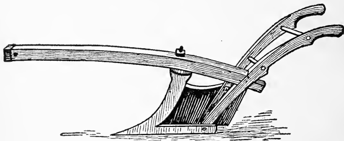
FIG. 32—THE NEWBOLD PLOW
