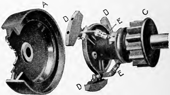
FIG. 332—CLUTCH
