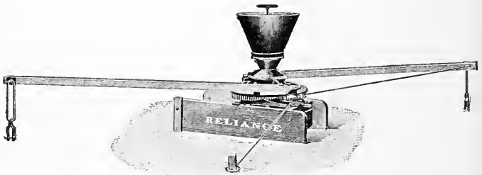
FIG. 177—A SWEEP MILL
