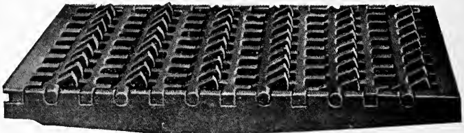
FIG. 222.—ROCKER GRATES
