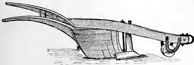
FIG. 31—WEBSTER'S PLOW
