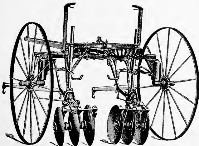
FIG. 70—A DISK CULTIVATOR
