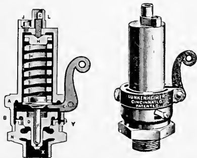
FIG. 236—POP VALVE
