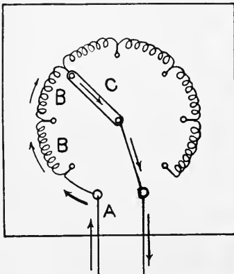
FIG. 348—PRINCIPLE OF RHEOSTAT
