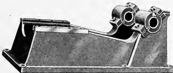
FIG. 291—BASE
