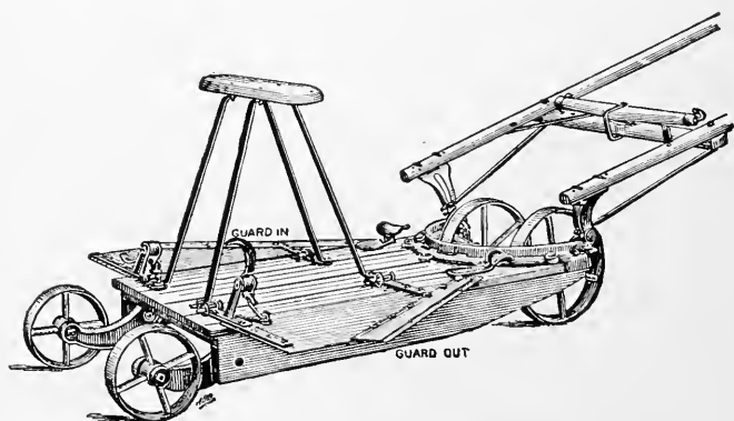
FIG. 116—A SLED CORN HARVESTER
