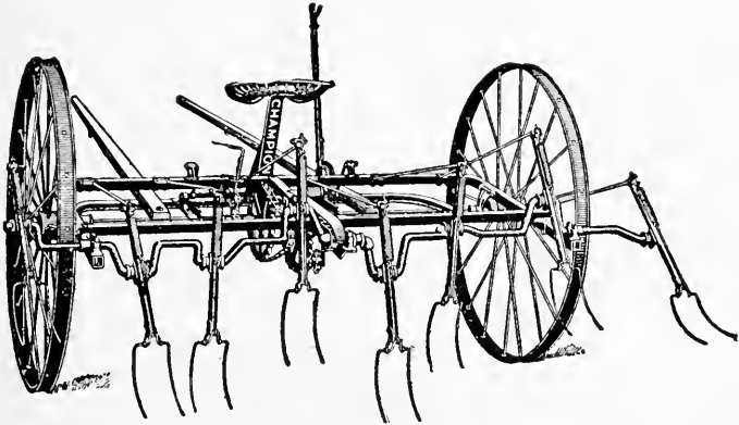
FIG. 128—AN EIGHT-FORK HAY TEDDER
