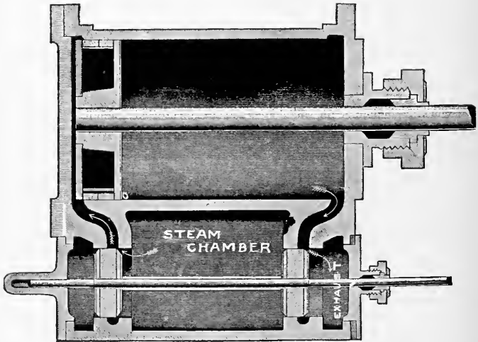
FIG. 254—PISTON VALVE
