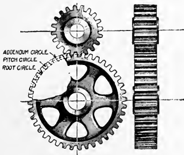
FIG. 24—SPUR GEARING
